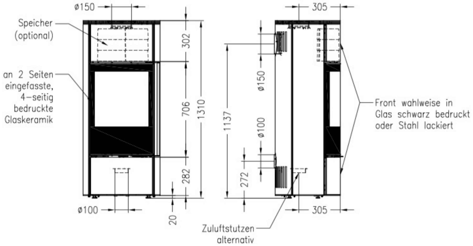
Vorderansicht M~1:20
